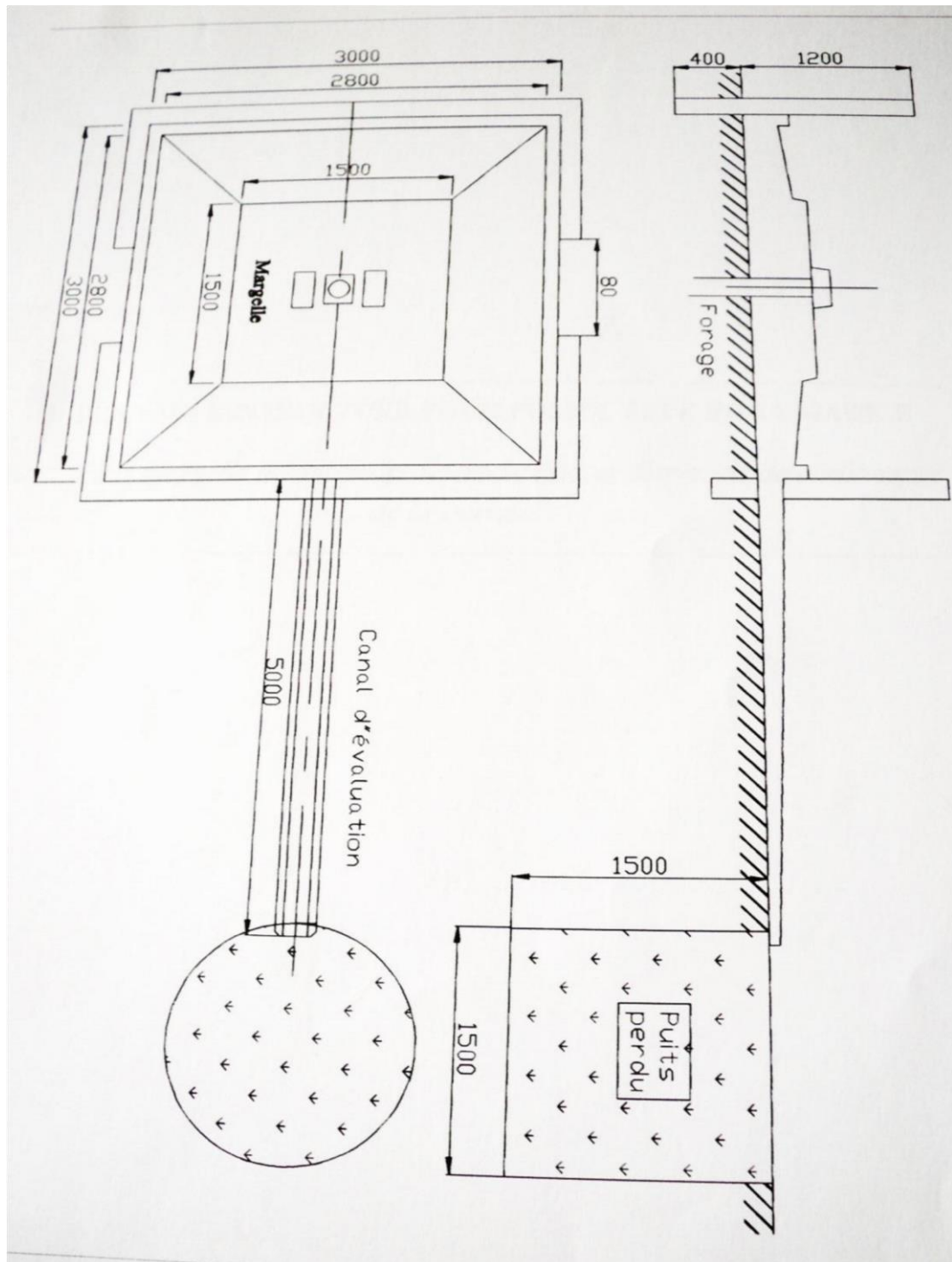
Schéma de la superstructure
